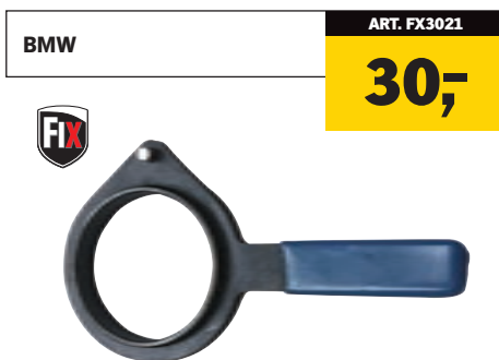
Distributie blokkeergereedschap incl. VANOS uitlijn gereedschap voor 1.8 en 2.0 benzine motoren (01-09).
